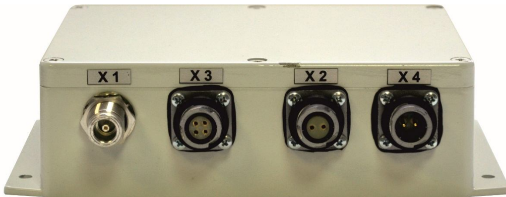
Рисунок 1.1.2.2 – Внешний вид приемника наведения ПСН-А со стороны левой боковой стенки изделия
