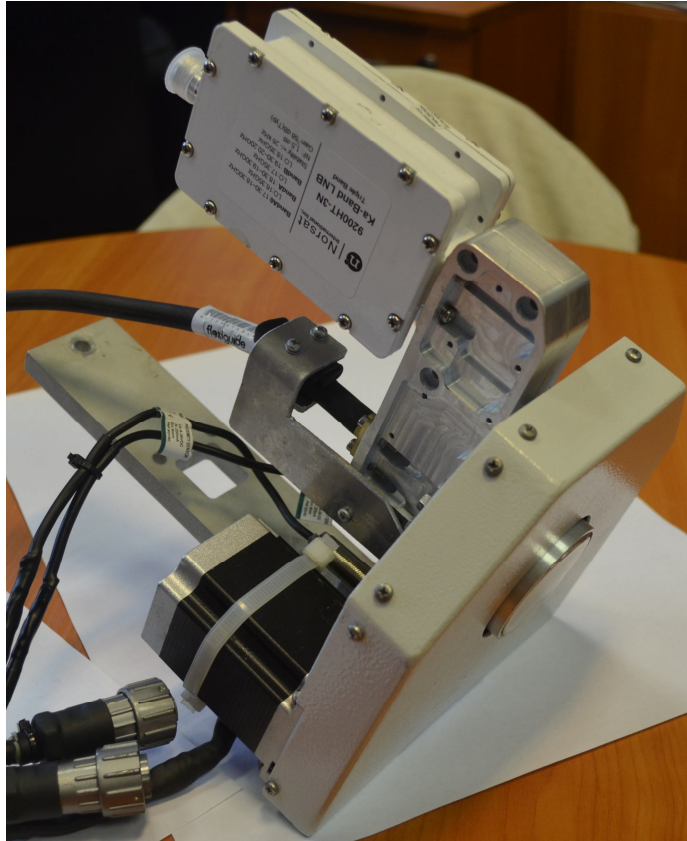
Рисунок 1.2.3 – Устройство вращения облучающим устройством ТИШЖ.301329.020
