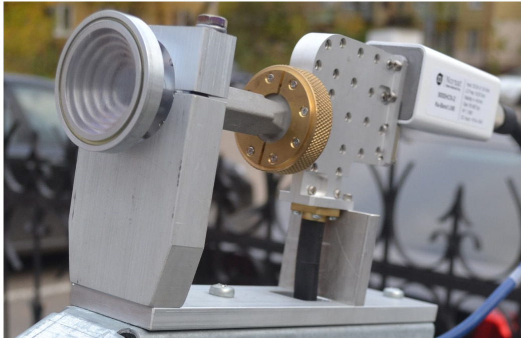
Рисунок 1.2.16 Внешний вид ОУ Ка-диапазона круговой поляризации
