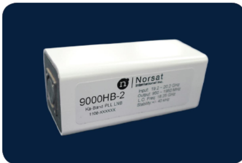
Рисунок 1.2.12 Внешний вид МШК 9000НСН-2
