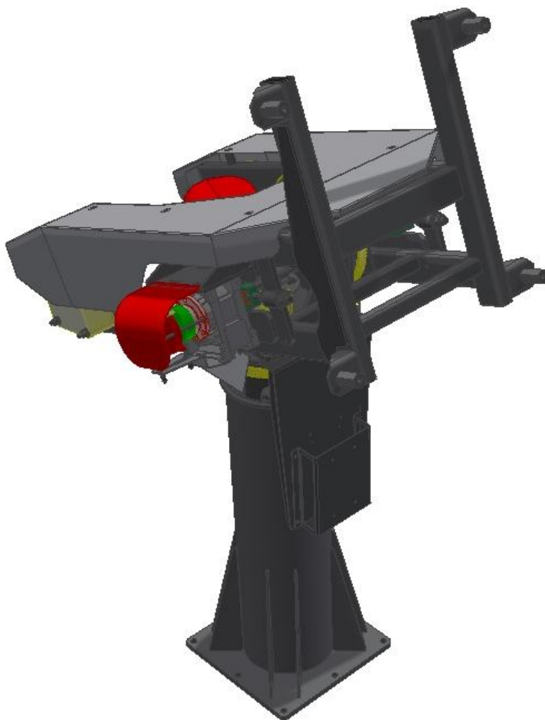
Рисунок 1.2.7 – Внешний вид опорно-поворотного устройства НПРК.464659.013
